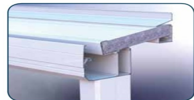
Detalle grueso 52 mm. Detail of 52 mm thickness Détail de l'épaisseur de 52 mm
